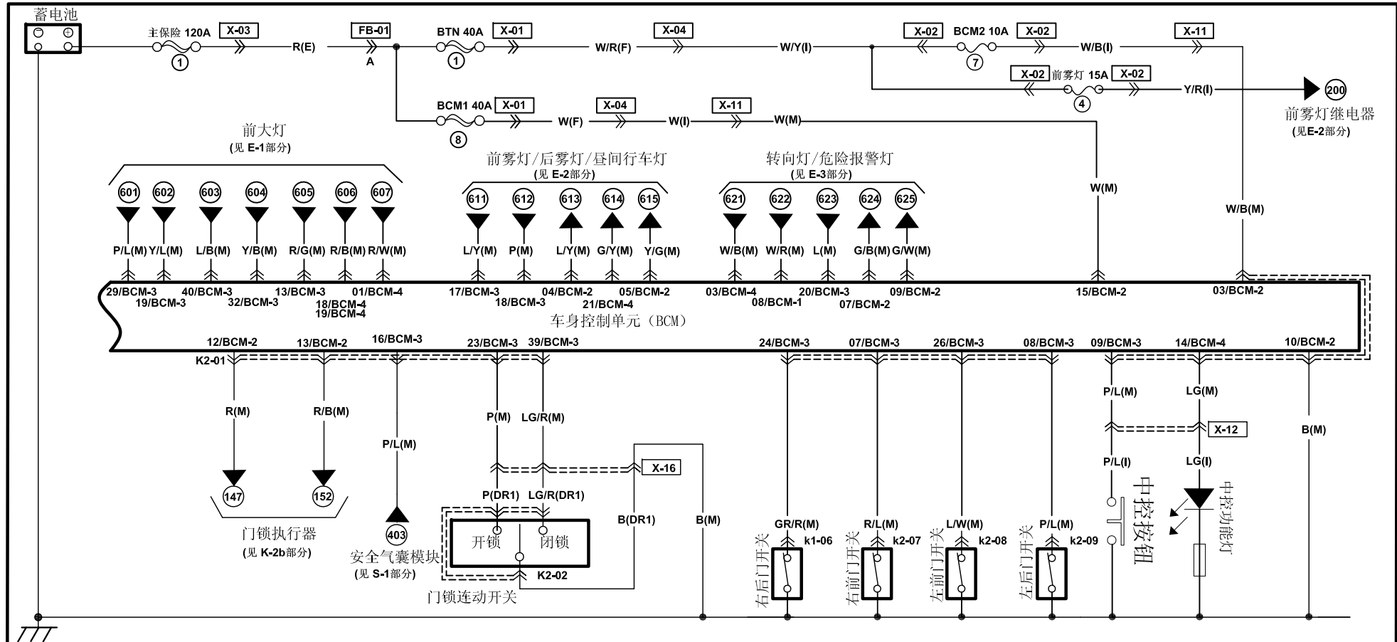
K2-02 门锁连动开关(DR1)
